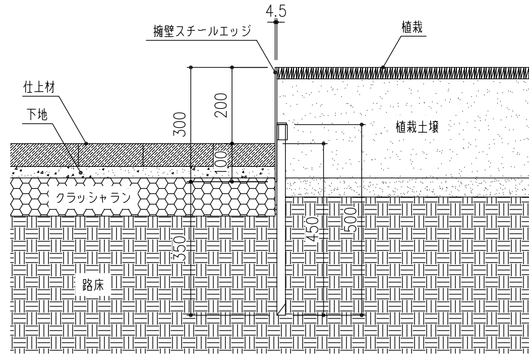
施工例 地盤強度 N値=3以上推奨
