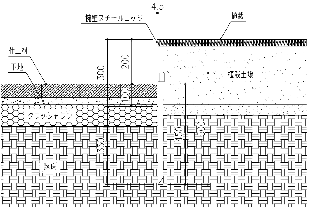
施工例
