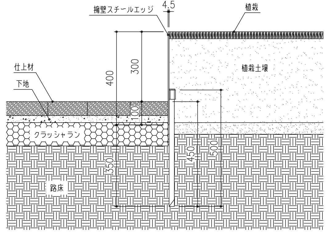
施工例
