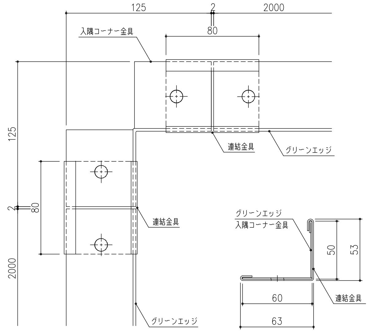
入隅コーナー連結図
