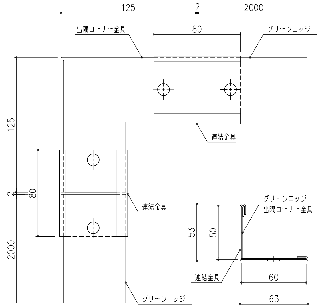
出隅コーナー連結図
