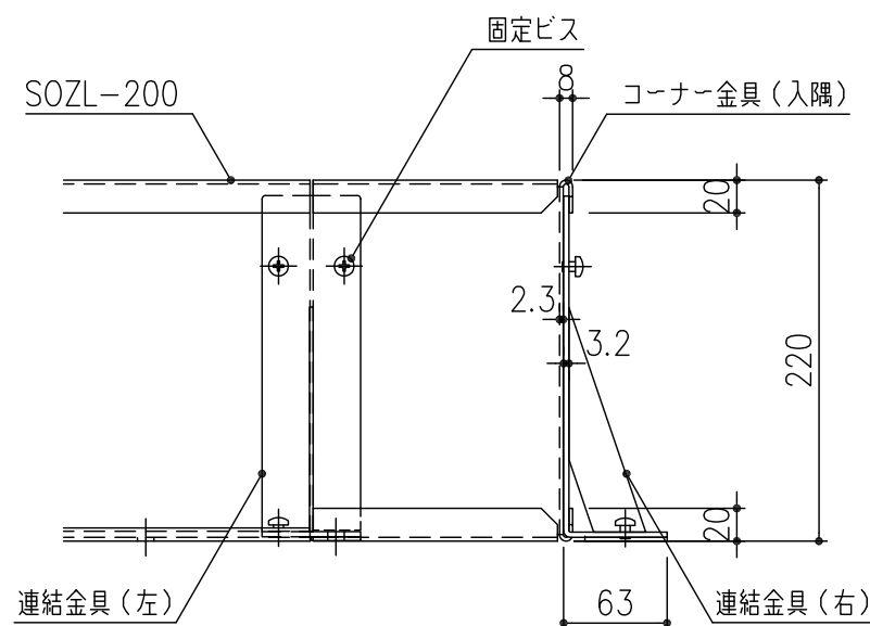
コーナー金具（入隅）
