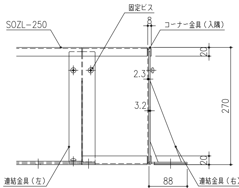
コーナー金具（入隅）
