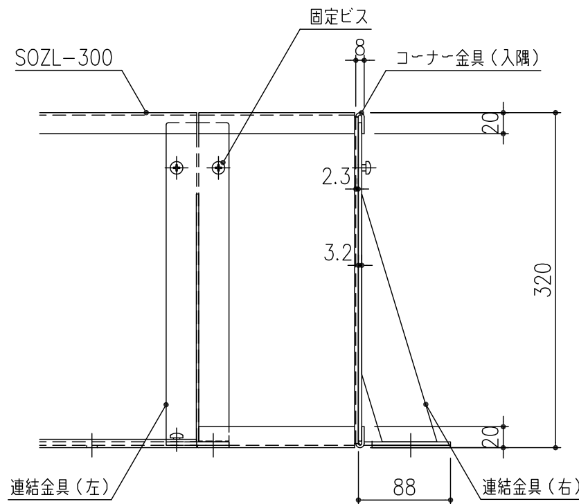
コーナー金具（入隅）
