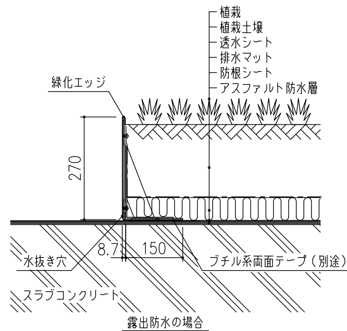
施工例図 S=1/10
