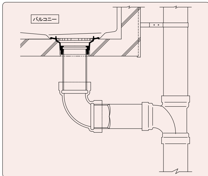
(図-2)枝配管による施工例
