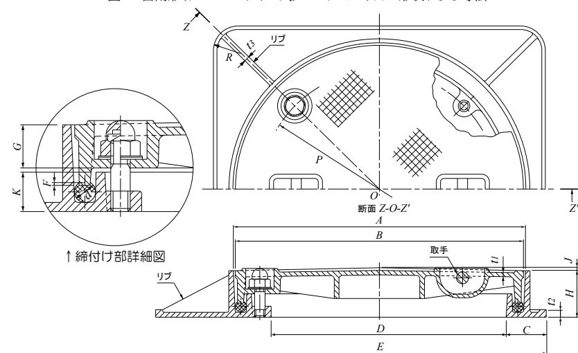
図2—密閉形（テーパー・パッキン式）マンホールふたの形状および寸法
