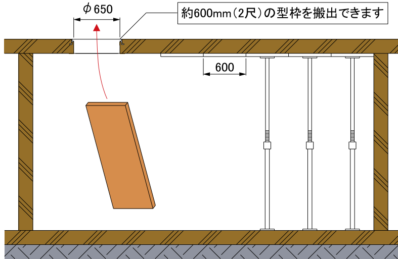
マンホールカバー 有効内径φ650リスト
