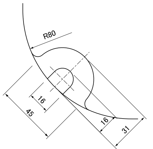
クサリ取付座詳細図
