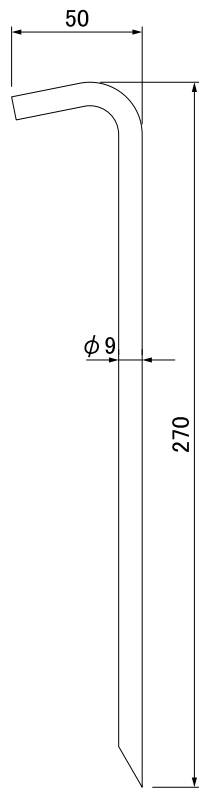
ペグ寸法図(参考)
