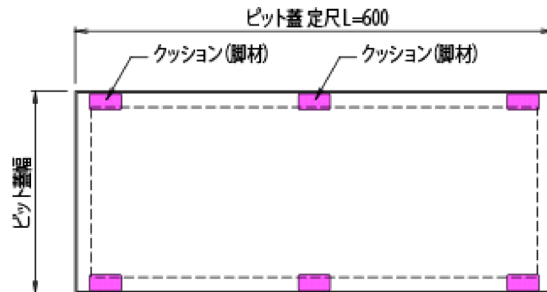
ピット蓋基本図
