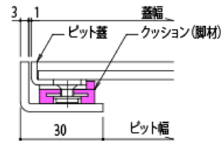
ピット蓋断面図
