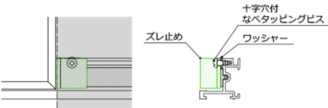
ズレ止め 例図
