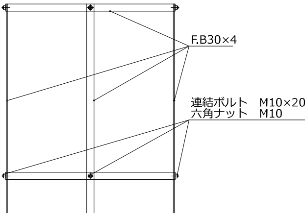
正面図
