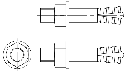
オールアンカー M12×70
